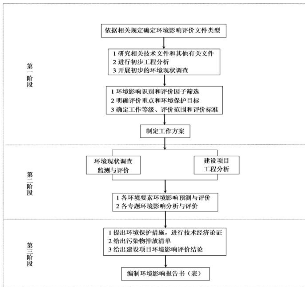
图 2.9-1 环境影响评价程序
