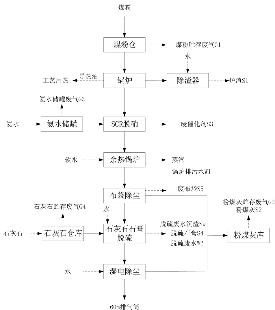
图 3.3-1 拟建项目生产工艺流程及产污环节
