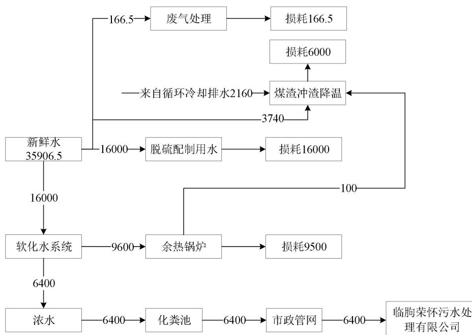
图3.2-3 拟建项目改建后水平衡图 (m³/a)
