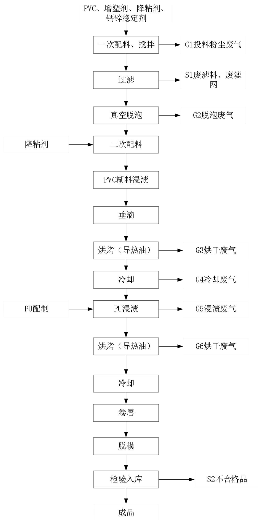
图3.1-3 手套生产工艺及产污环节流程图
