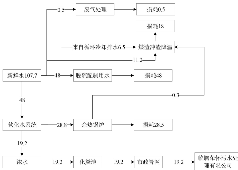
图3.2-2 拟建项目改建后水平衡图 (m³/d)
